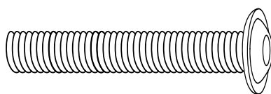
Flanschkopfschraube 8x50 mm für Holzkufe Flange head screw 8x50 mm for wooden runner
