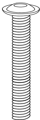
Flanschkopfschraube 8x50 mm für Holzkufe Flange head screw 8x50 mm for wooden runner
