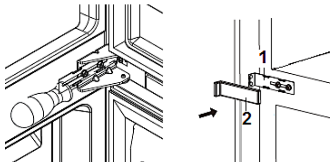
1: Mittlere Klammer; 2: Abdeckung für mittlere Klammer
