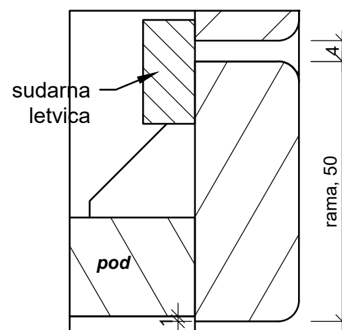
Detalj:X (1:1)
