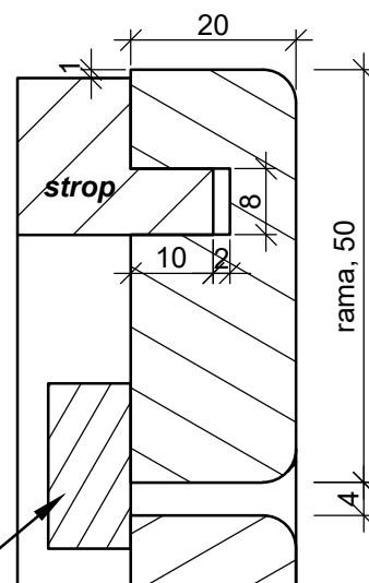
Detalj:F (1:2)
