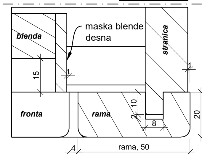
Detalj:C (1:1)
