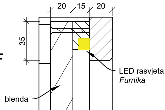
Detalj:X (1:1)
